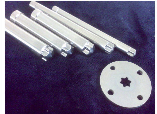
Werkstoff: HSS 1.3343
