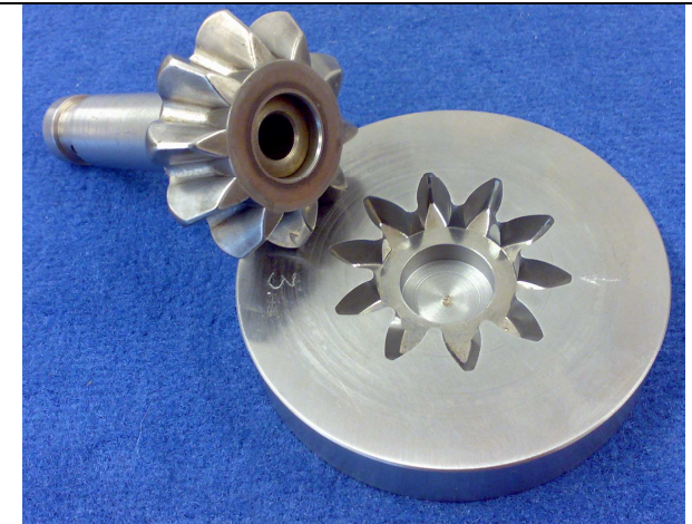
Werkstoff: ASP2012
